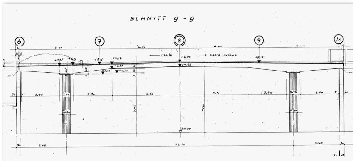
Abbildung 4: Bauwerksplan Grüne Brücke (Bestand)
