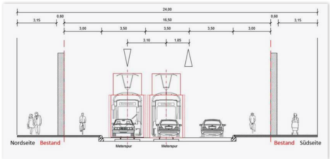
Abbildung 5: Mögliche Aufteilung des Verkehrsraums unter der Grünen Brücke
